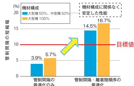
● 管制間隔の短縮効果を確認 （羽田空港を模擬したシミュレーション）
