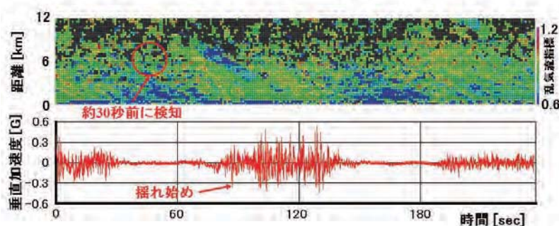
● 晴天乱気流の検知例
